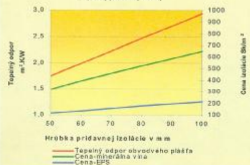
Zateplenie obvodového plášťa z plnej pálenej tehly
